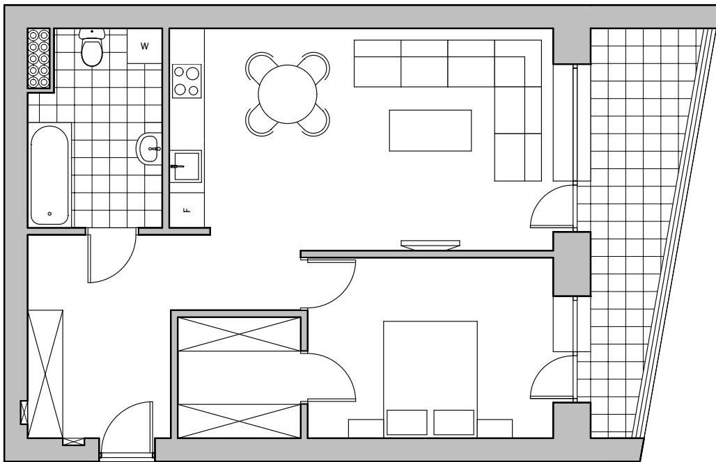
BUTO PLANAS PRIEŠ REKONSTRUKIJĄ
